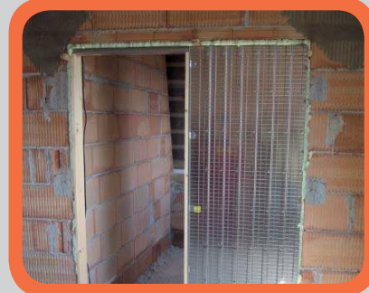
Zapěněné pouzdro ve stavebním otvoru
